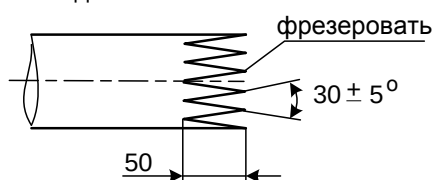
Эскиз обработки края звукотода для монтажа АР-11
