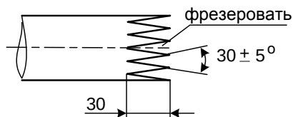
Эскиз обработки края звукотода для монтажа АР-13
